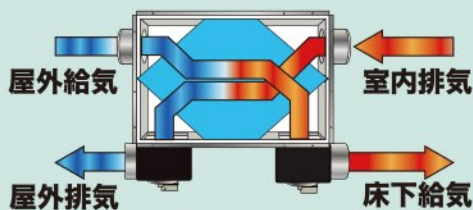
2 8 全熱交換器
