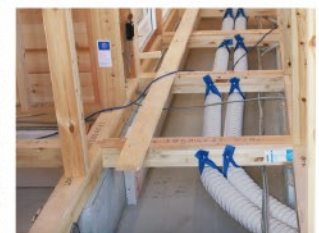
床下配管
